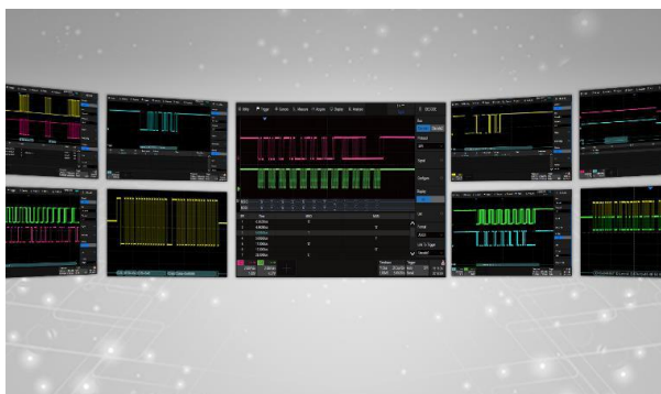
Логический анализатор (16 каналов), для работы в режиме MSO необходимы программная опция SDS6000Pro-16LA и логический пробник SPL2016 (на фото - слева).
